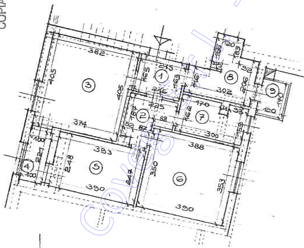
PIANTA APPARTAMENTO PIANO 5° N° 48 SC. 1/100
